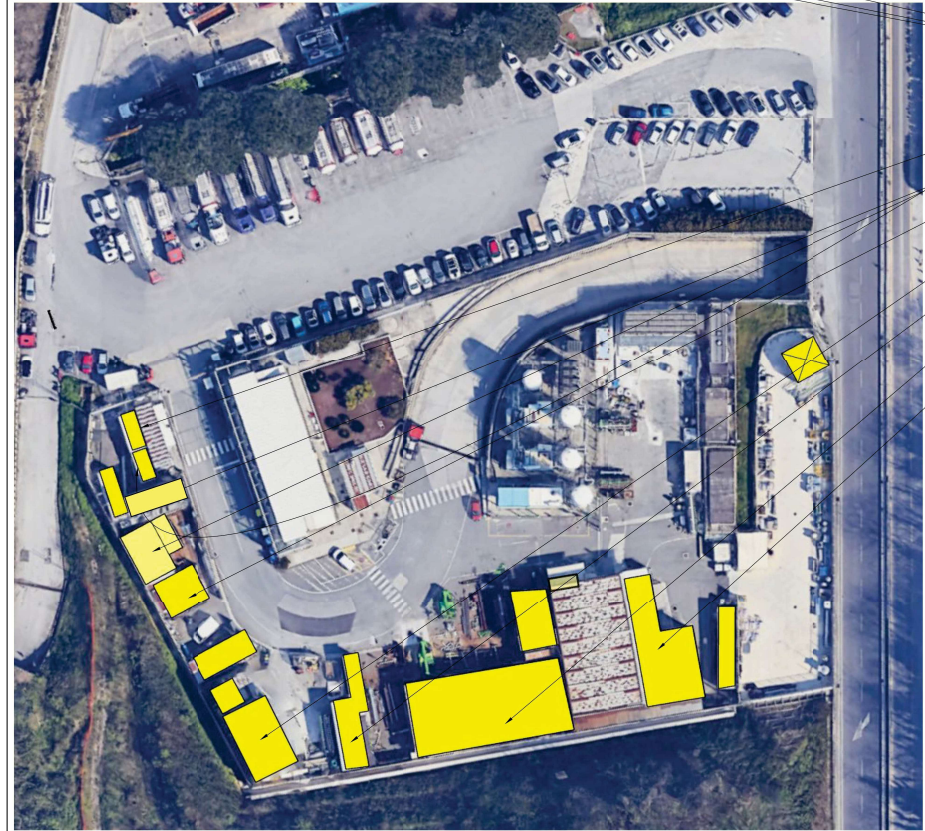
FOTOGRAFIA ZENITALE DELL' "AREA NORD" INFINEUM CON EVIDENZIATI GLI EDIFICI ESISTENTI PREVISTI IN DEMOLIZIONE
